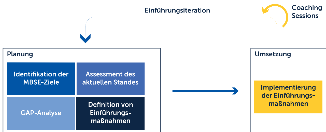
Abbildung 6: MBSE-Einführungsprozess
