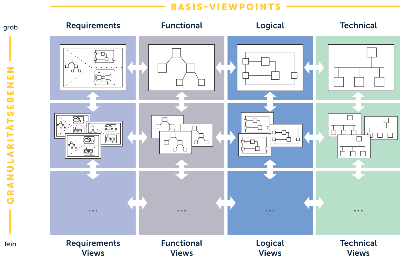
Abbildung 4: SPES-Matrix
